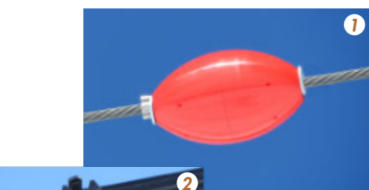
▲ Un floteur OGM pour visualiser les câbles.
