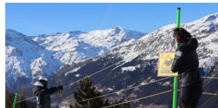
À Val Cenis, le choix s'est porté sur des piquets polycarbonates verts, support de quatre rangs de corde élastique sur lesquels sont installés des fanions souples et des panneaux d'avertissement de la boîte à outils du plan d'actions en faveur du Tétrasylyre (PATLY). Cette matérialisation semble idéale car bien respectée.
