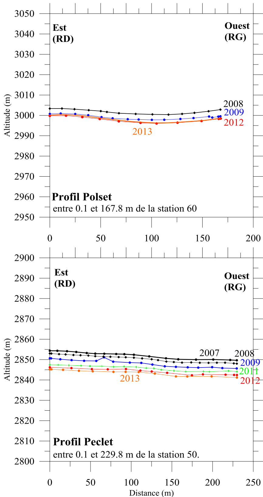
Figure 5a : Variations d'altitude aux profils Polset (3000 m d'altitude) et Peclat (2850 m d'altitude). La situation de ces profils est reportée sur la figure 1. RD et RG signifient Rive Droite et Rive Gauche.
