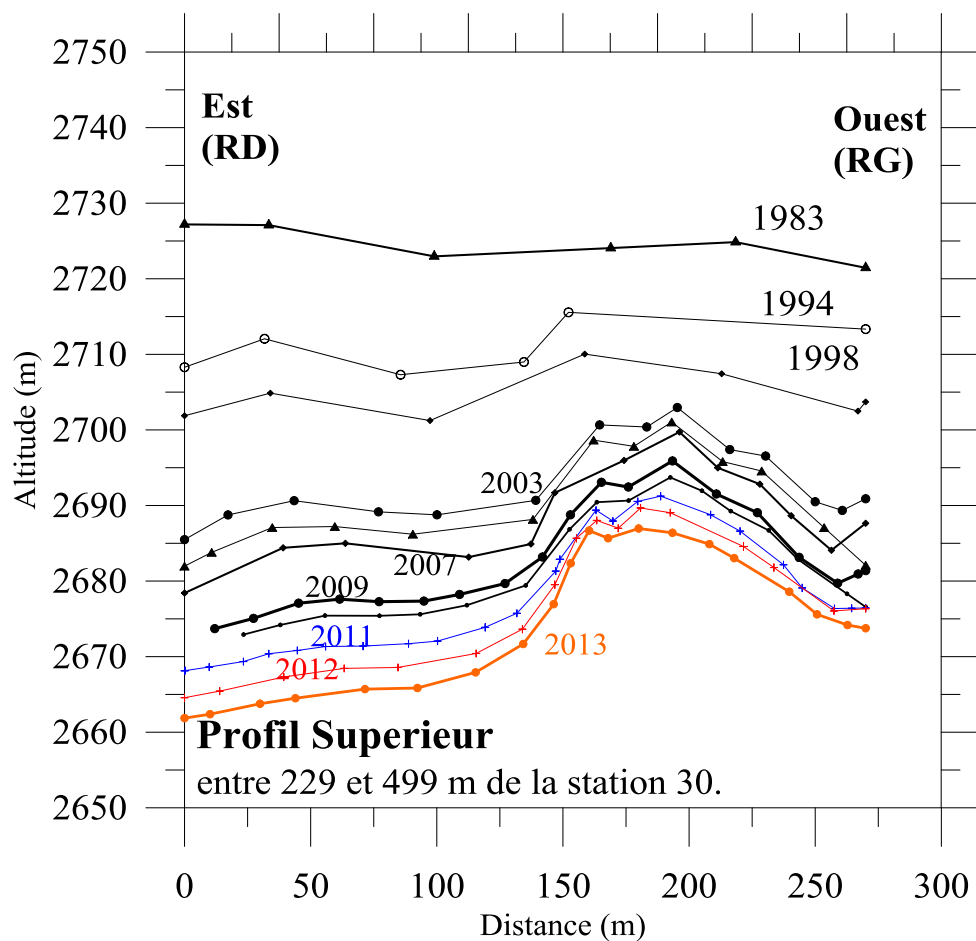
Figure 5b : Variations d'altitude aux profils Suprême et Supérieur (profils vus de l'aval). La situation de ces profils est reportée sur les figures 1 et 7. RD et RG signifient Rive Droite et Rive Gauche.
